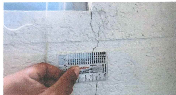
SECRETARÍA ACADÉMICA Y VOLUNTARIADO (GRIETAS EN MUROS)
