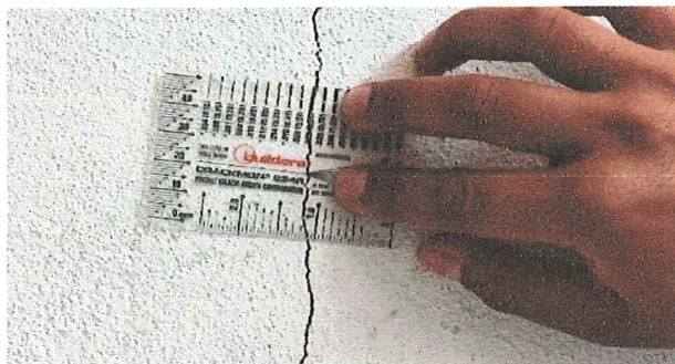
DIRECCIÓN DE BIBLIOTECAS (GRIETAS VERTICALES)
