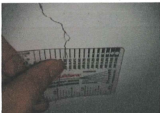
EDIFICIO CEDA (VIGAS Y COLUMNAS DE CONCRETO CON LOSA MACIZA)
