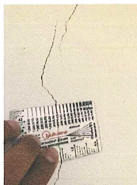
CENTRO DE REHABILITACIÓN (SALA DE LA LAGUNA) (GRIETAS EN MUROS EXTERIORES)
